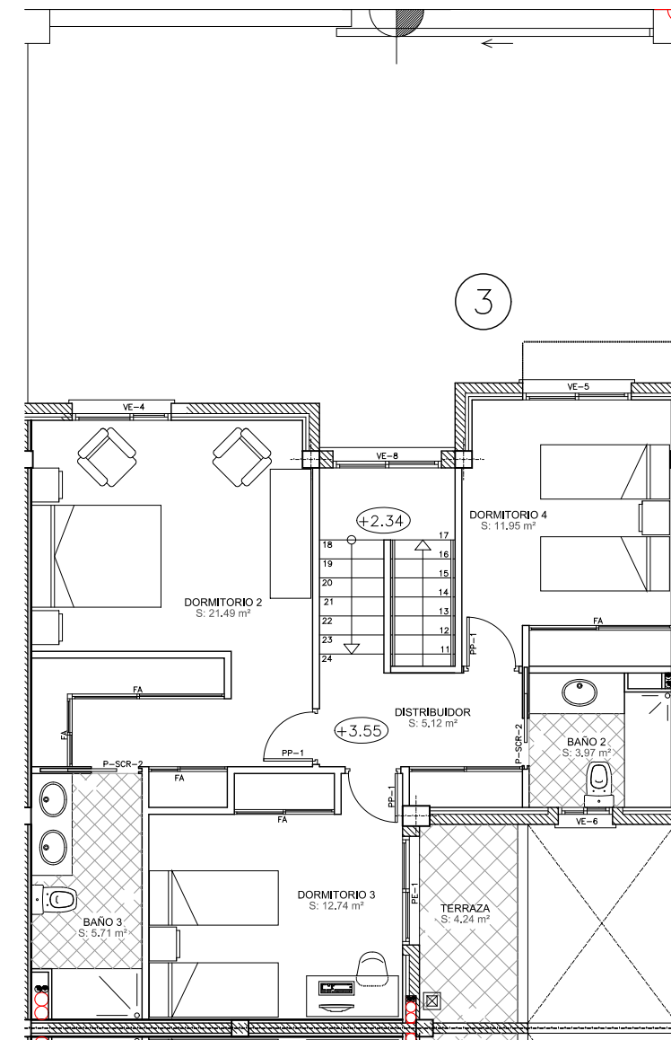
PLANTA PRIMERA
