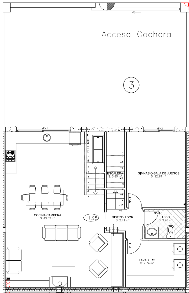
PLANTA SÓTANO
