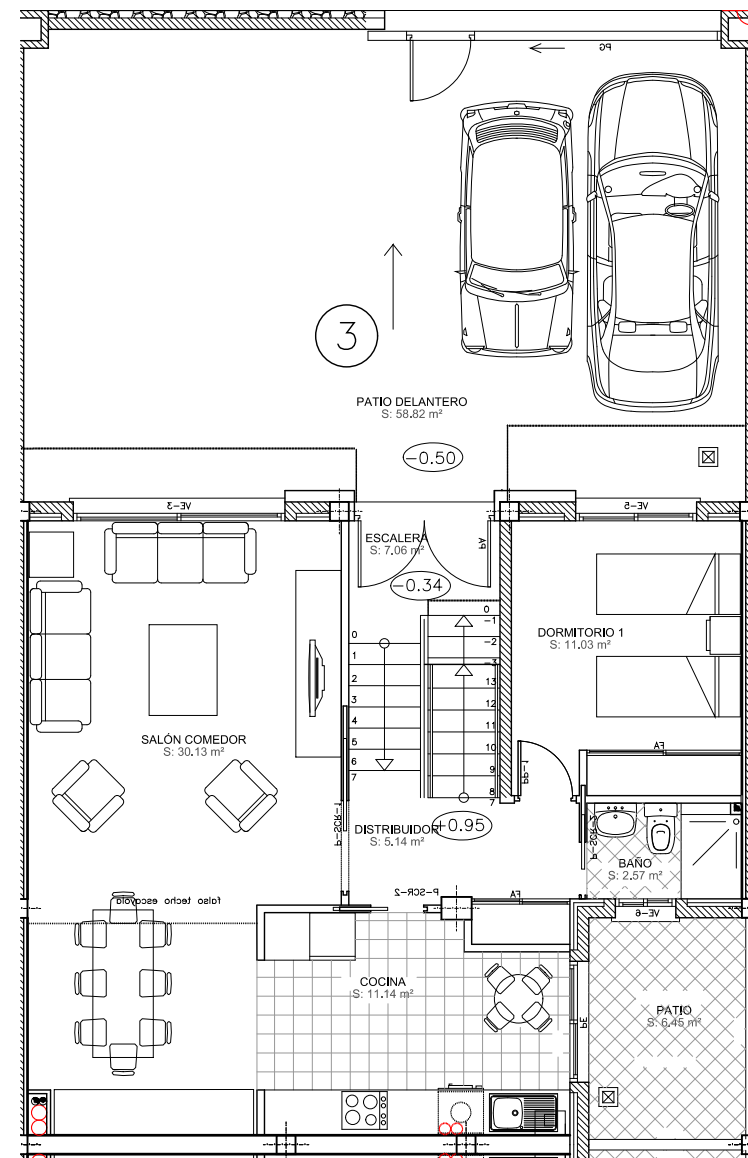
PLANTA BAJA
